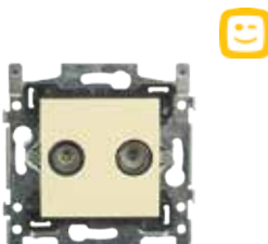
EDB 02 CRÈME (RAL 1013) TV/FM WANDCONTACTDOOS MET AFDEKPLAAT Art. nr. 695 021 172
